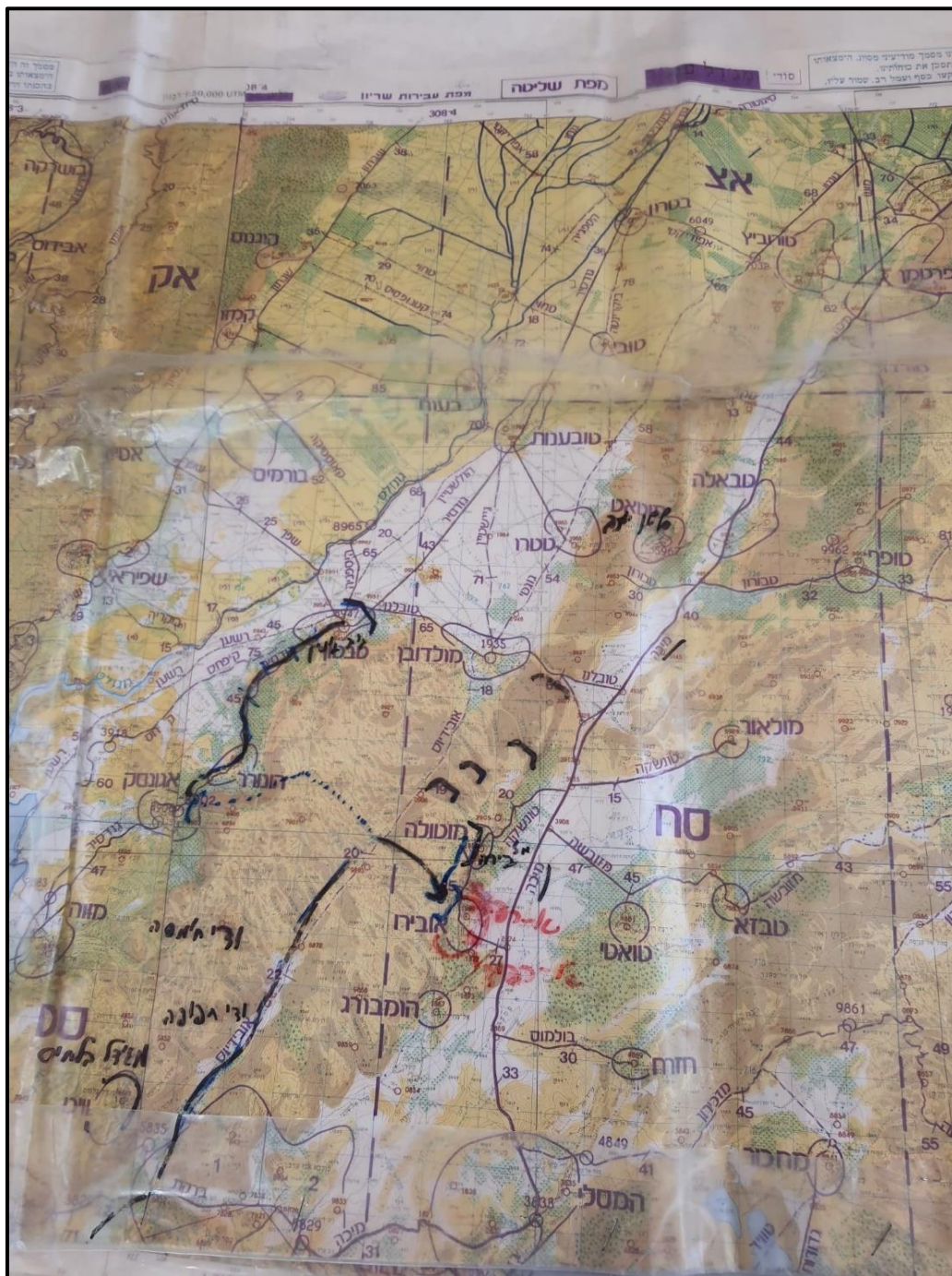
מפת שליטה 'הוריקן' של אזור ארפיז 27
