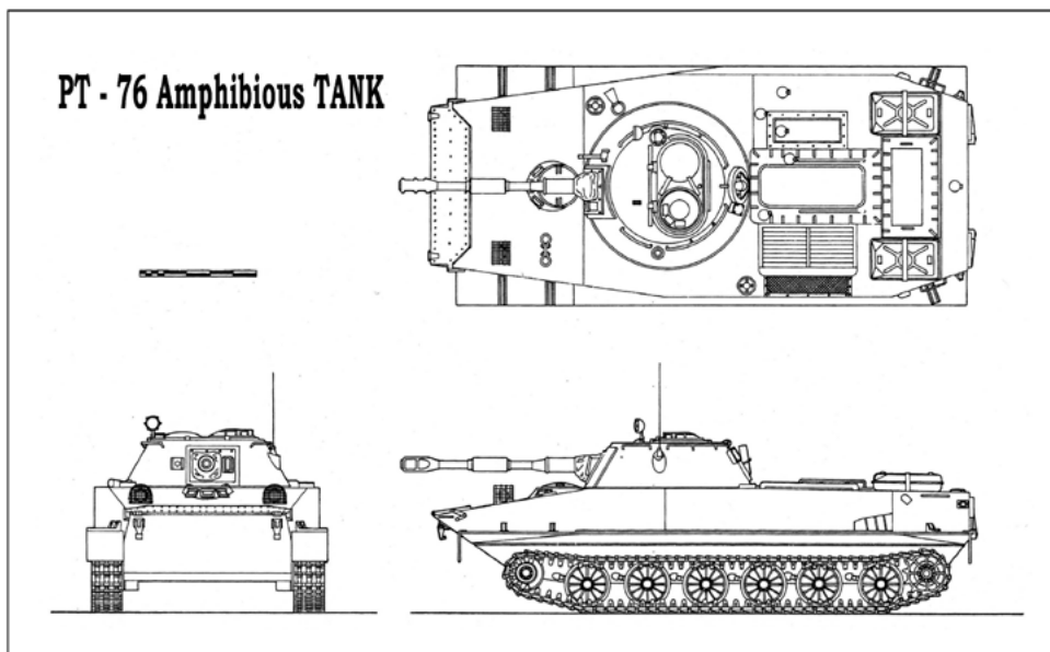
פי-טי-76 – טנק אמפיבי 29
