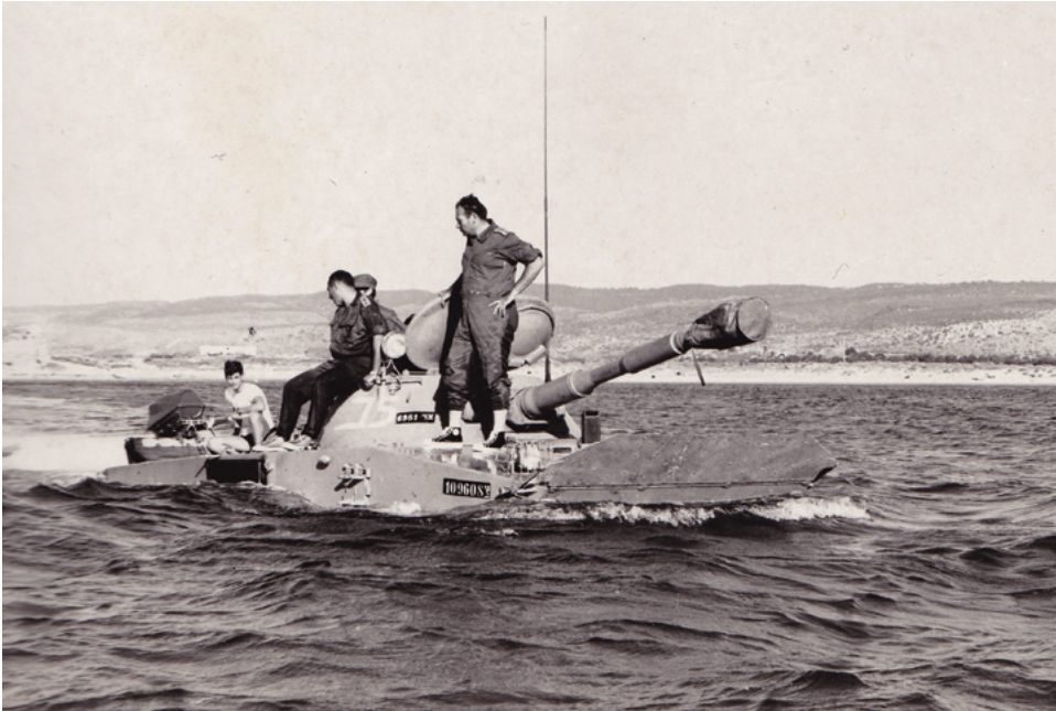
ניסוי הישט עם טנק פי-טי-76 על ידי מדור הישט בתח"ש, 1970. ראש המדור, יואל גונן, עומד על הסיפון מימין (ארכיון אמנון טישלר, צילום: גי"ש-תח"ש).
