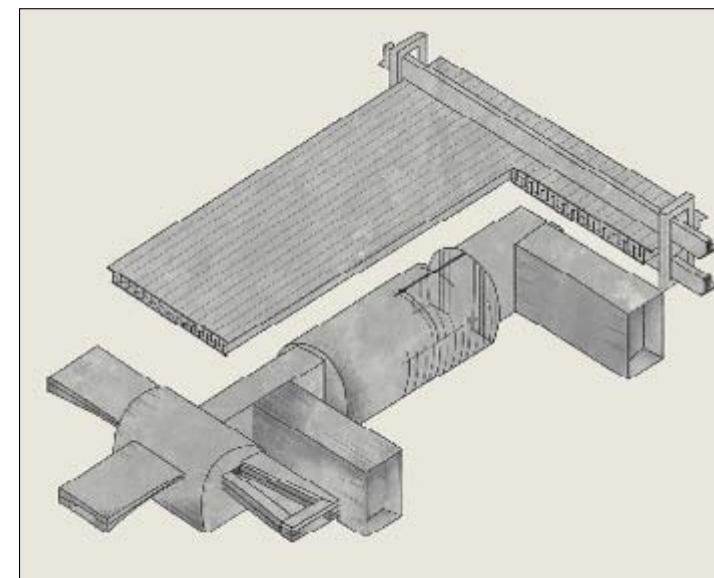
תרשים בונקר במוצבי התעלה - בבונקר חדר שהייה ועמדת ירי; מעליו יש שכבות הגנה ובהן עפר ושכבת פיצוץ
