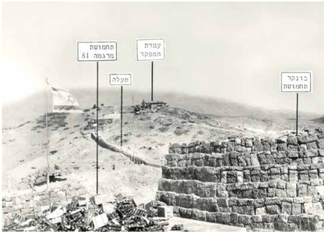
למעלה: מוצב 104 ברמת הגולן - תעלת קשר היקפית ועמדות לחימה מימין: תרשים מוצב 104
